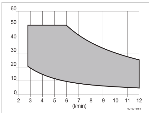
Fig. 27 Modelo 12 litros
