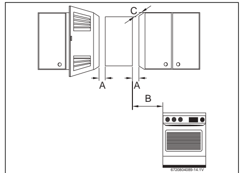
Fig. 19 Distancias mínimas
