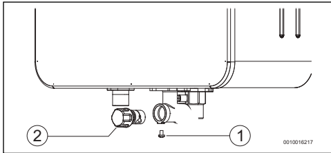
Fig. 15 Purga
